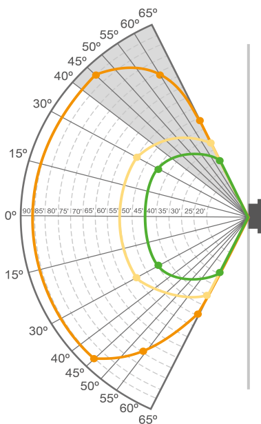
Figura 3 Campo visivo per l'eptano
