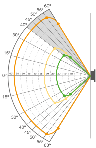
Figura 6 Campo visivo per il propano
