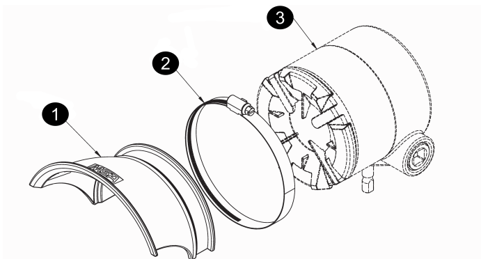
Figura 20 Vista esplosa
