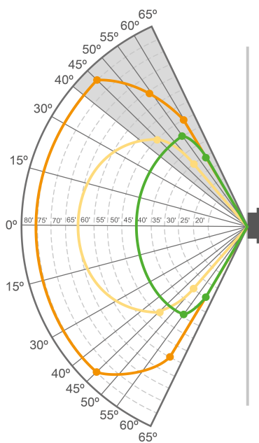
Figura 4 Campo visivo per il metano
