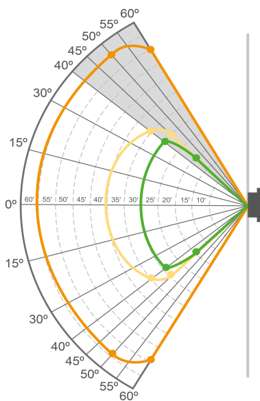
Figura 7 Campo visivo per l'etano
