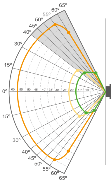
Figura 9 Campo visivo per l'idrogeno dell'FL500-H 2 in orizzontale
