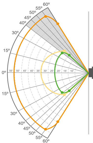
Figura 8 Campo visivo per il butano
