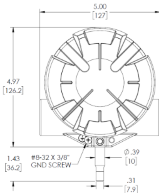
Figura 10 FL500 - Panoramica - Vista anteriore
