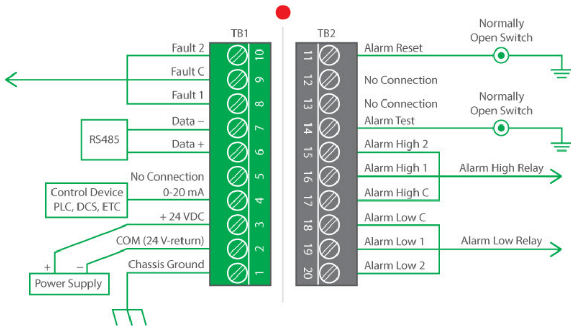
Figura 16 Schema di cablaggio
