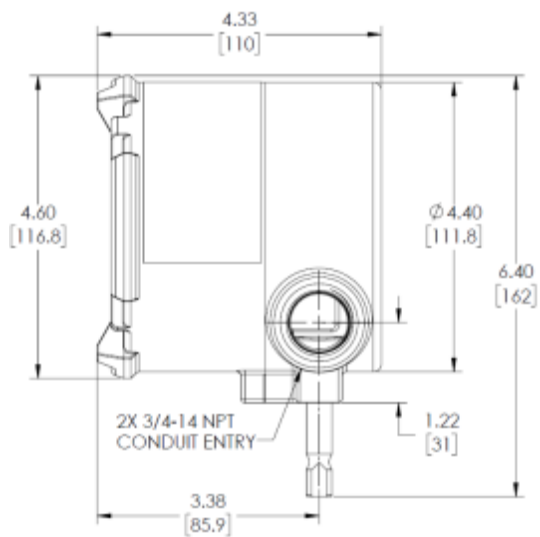
Figura 11 FL500 - Panoramica - Vista posteriore
