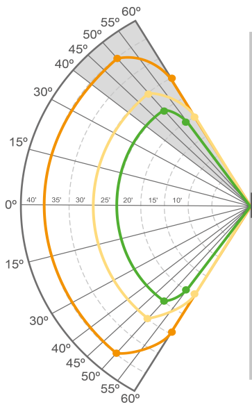
Figura 5 Campo visivo per il metanolo
