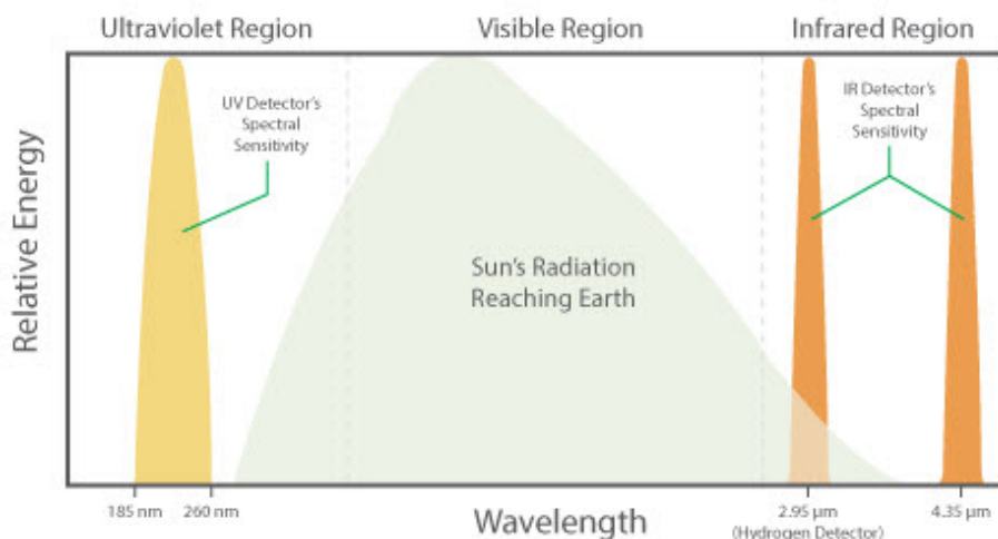
Figura 1 Riposta spettrale dei rilevatori di radiazioni UV e IR
