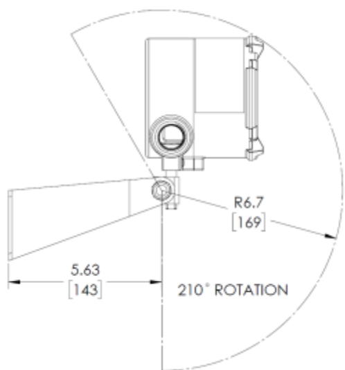
Figura 12 FL500 e staffa di montaggio - Vista laterale
