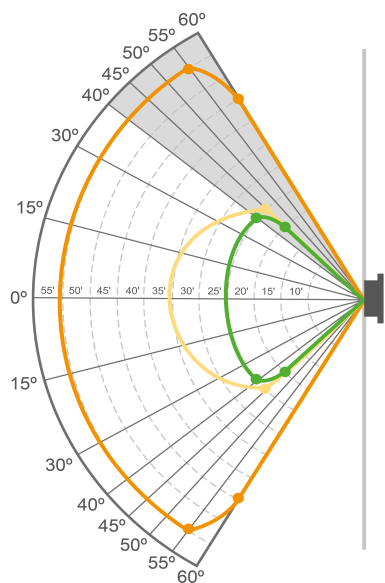
rysunek8 Pole widzenia butanu
