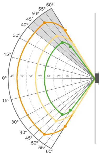
rysunek5 Pole widzenia dla metanolu
